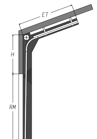
Наклонный высокий тип монтажа с верхним расположением вала
