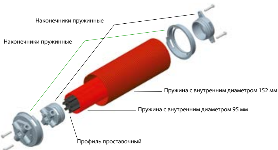
СХЕМАТИЧЕСКОЕ ИЗОБРАЖЕНИЕ ДУПЛЕКСНОЙ ПРУЖИНЫ
