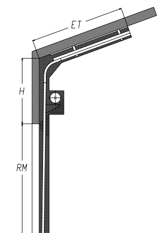
Наклонный высокий тип монтажа с нижним расположением вала
